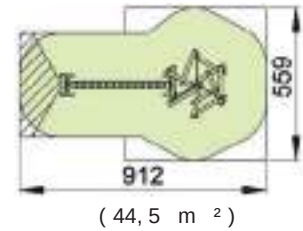
S820 - M i k a d o w i t h w i g g l e w a g g l e
